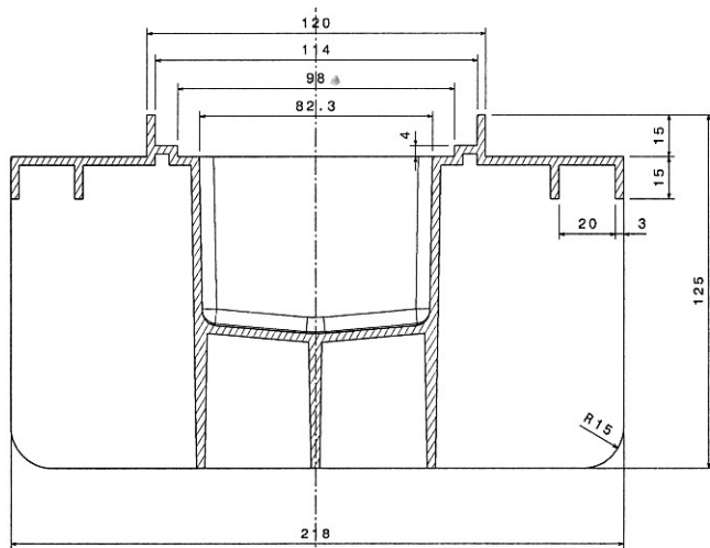
Vista in sezione B-B Scala: 1:1
