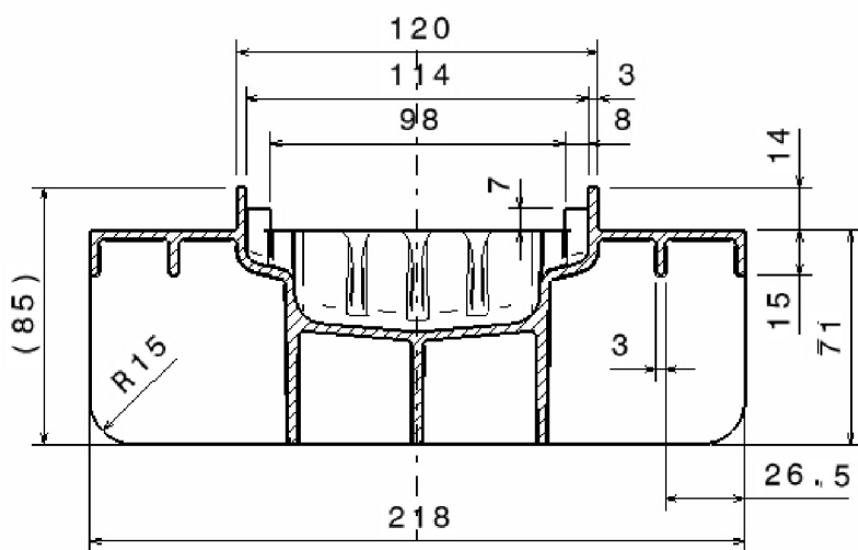
Vista in sezione B-B Scala: 1:2
