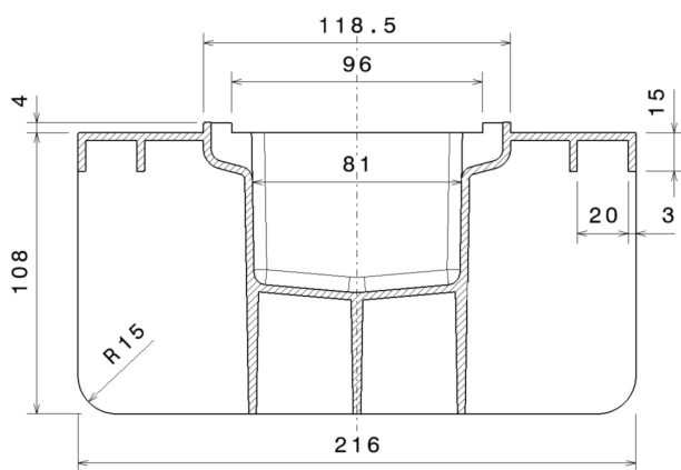
sezione B-B
